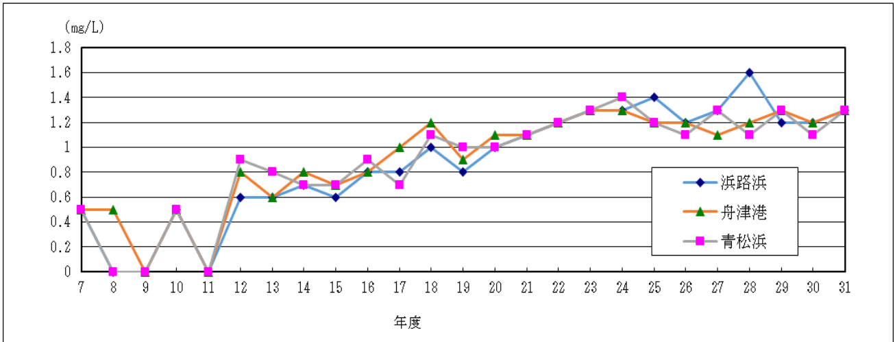
図1 湖南3地点のCOD推移
