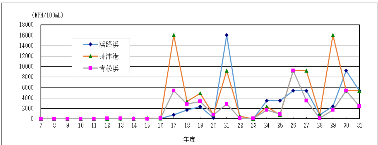
図3 湖南3地点の大腸菌群数（最大値）の推移
