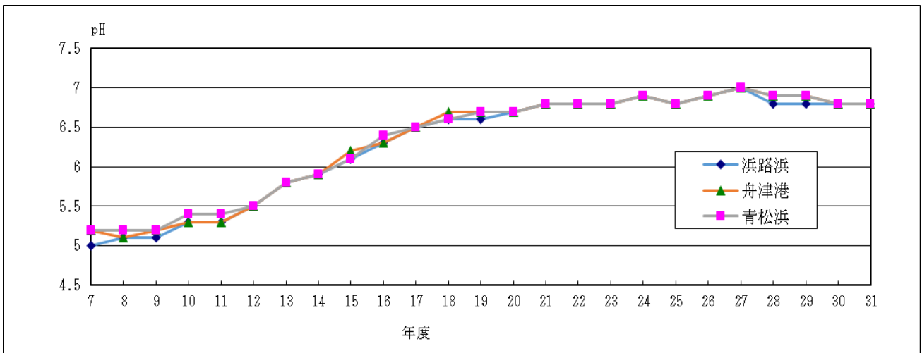
図2 湖南3地点のpH推移
