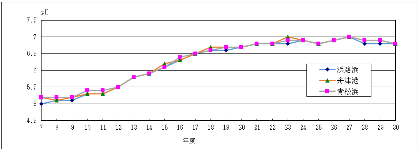
図2 湖南3地点のpH推移
