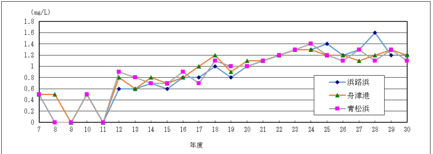
図1 湖南3地点のCOD推移
