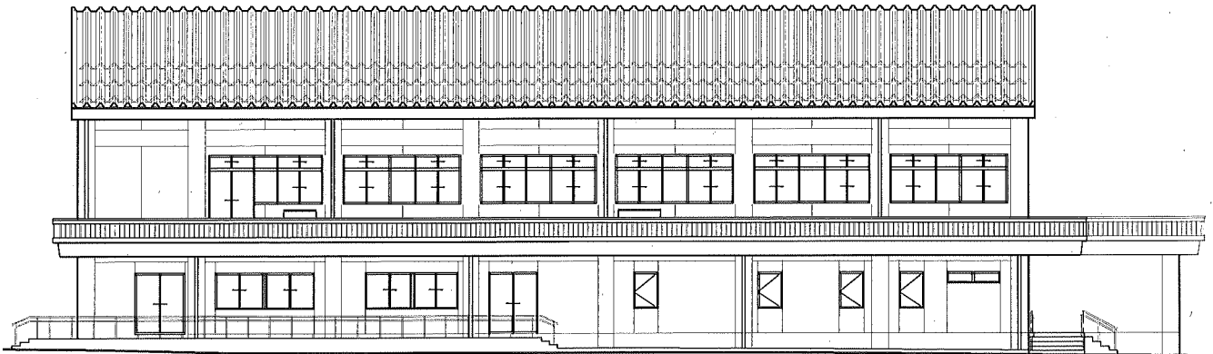
南側立面図
