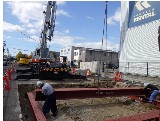
桁受設置状況
