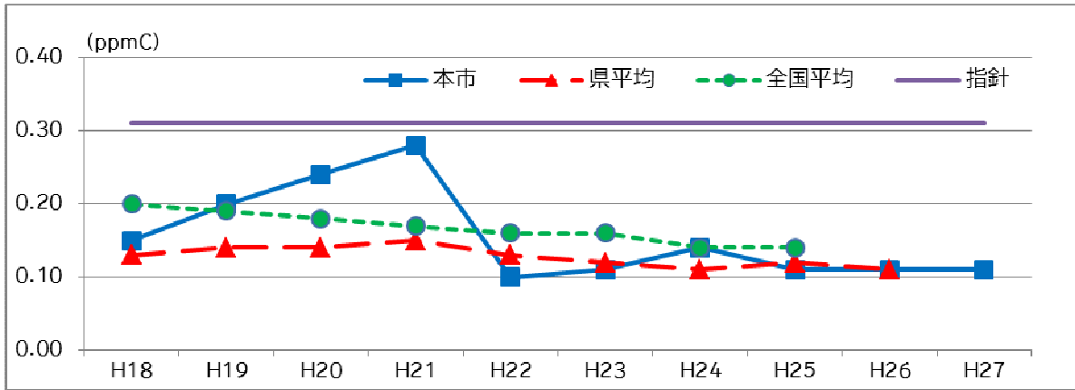
図 6 非メタン炭化水素濃度 (午前 6 時～9 時の 3 時間平均値の年平均値) の推移
