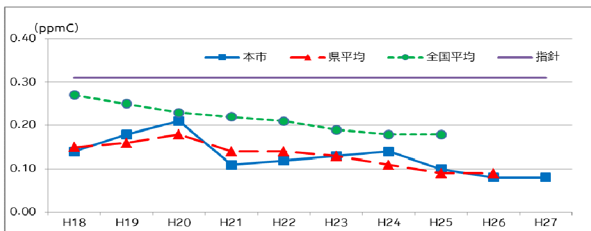
図11 非メタン炭化水素濃度 (午前6時~9時の3時間平均値の年平均値) の推移
