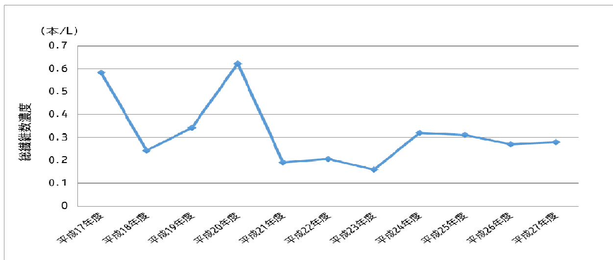
図1 一般環境大気中アスベスト濃度調査結果
