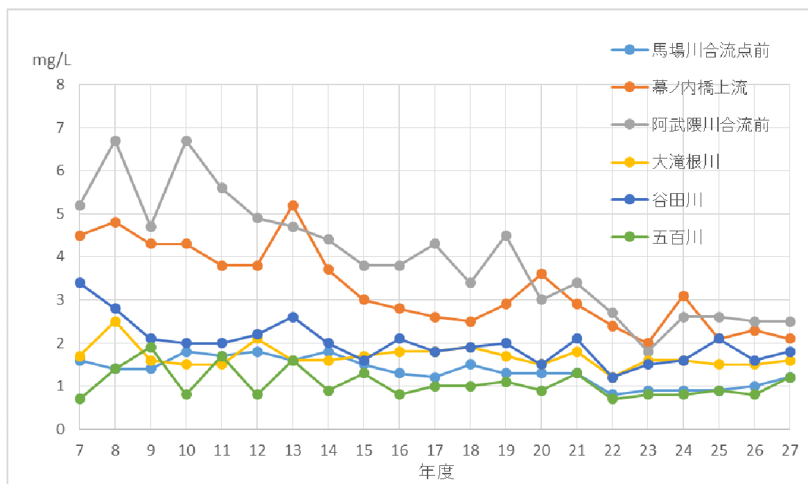
図1 河川のBOD値の推移
