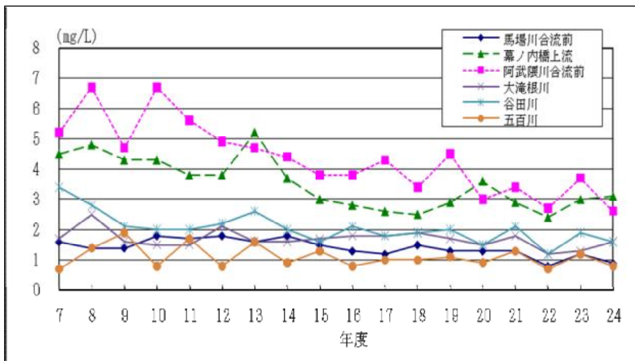
図-1 河川のBOD値の推移
