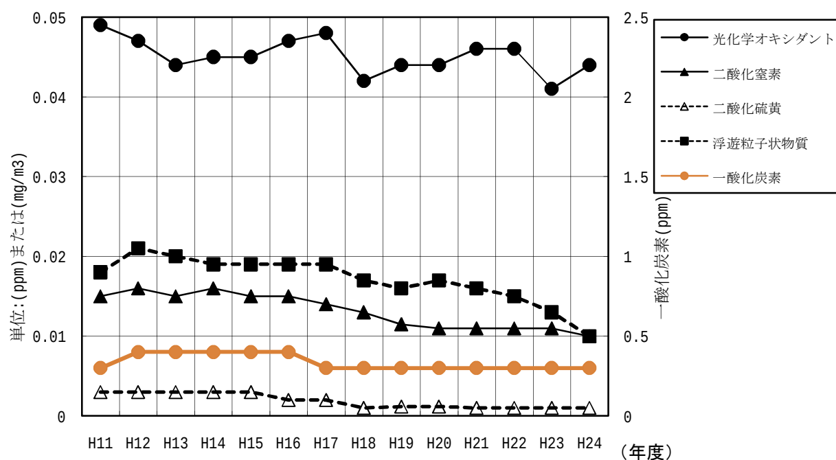
図1 大気汚染の経年変化(市内7局の年平均値)
