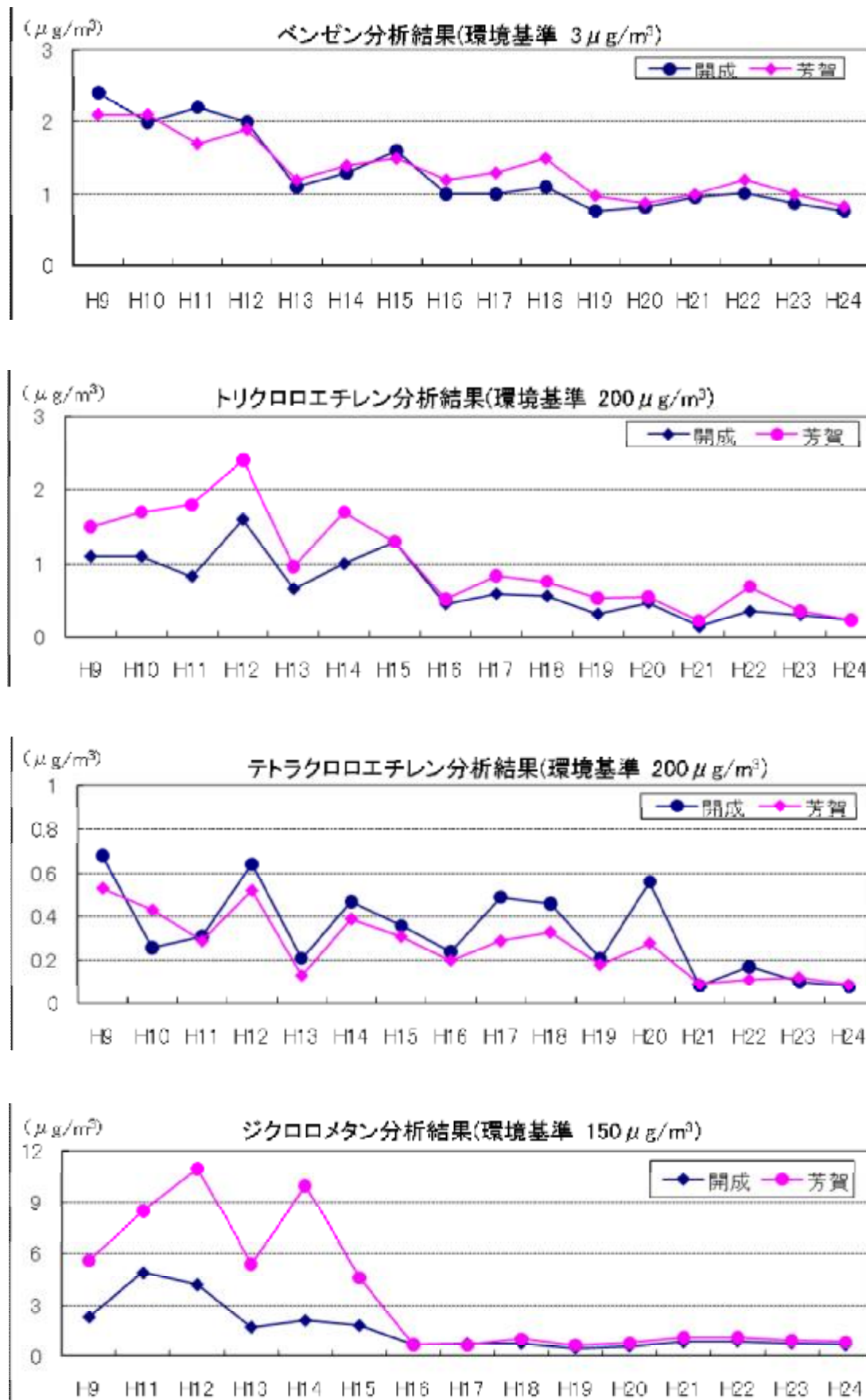
図1 有害大気汚染物質の推移
