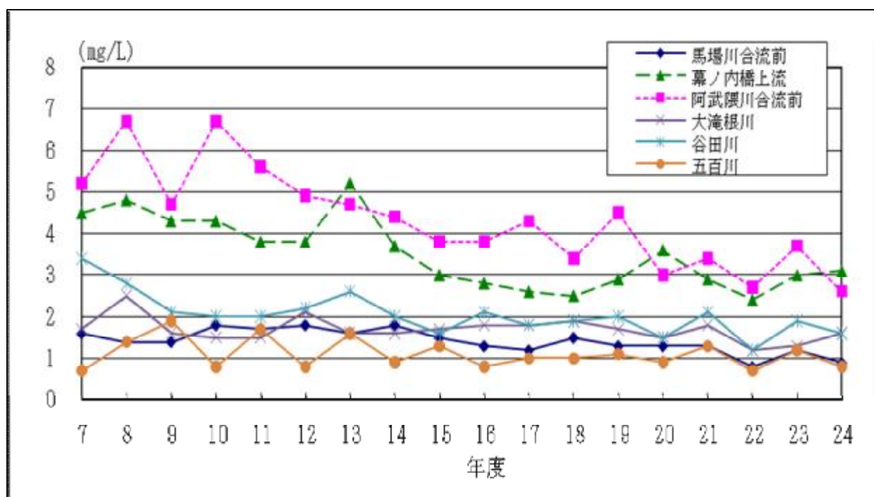
図－１ 河川のＢＯＤ値の推移
