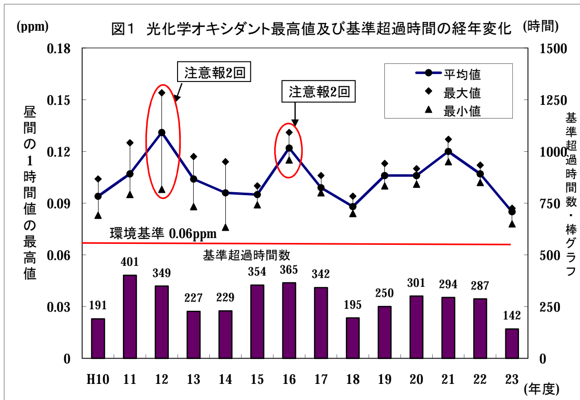
図2 光化学オキシダントの環境超過時間数と最高濃度の推移
