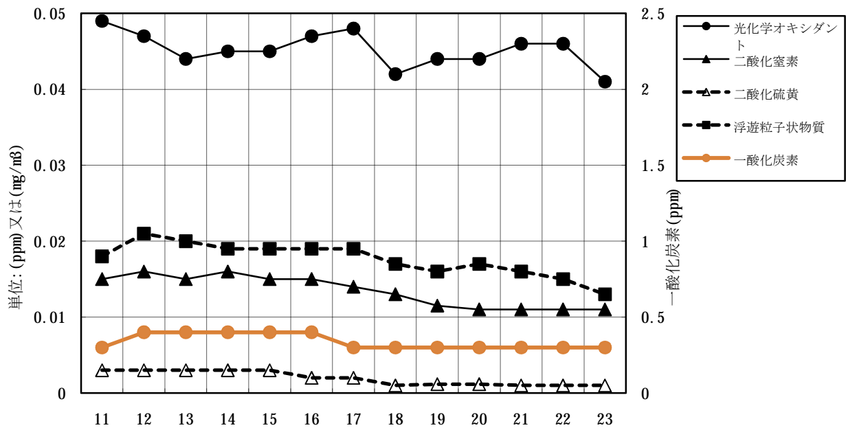
図1 大気汚染の経年変化（市内7局の年平均値）
