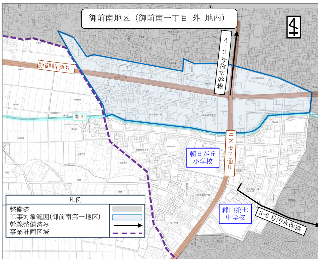
図 1-1 御前南第一地区（概要図）
