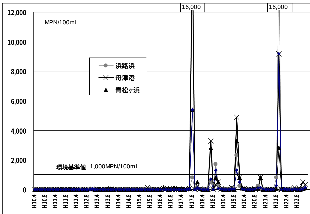
図－３ 湖南３地点の大腸菌群数の推移
