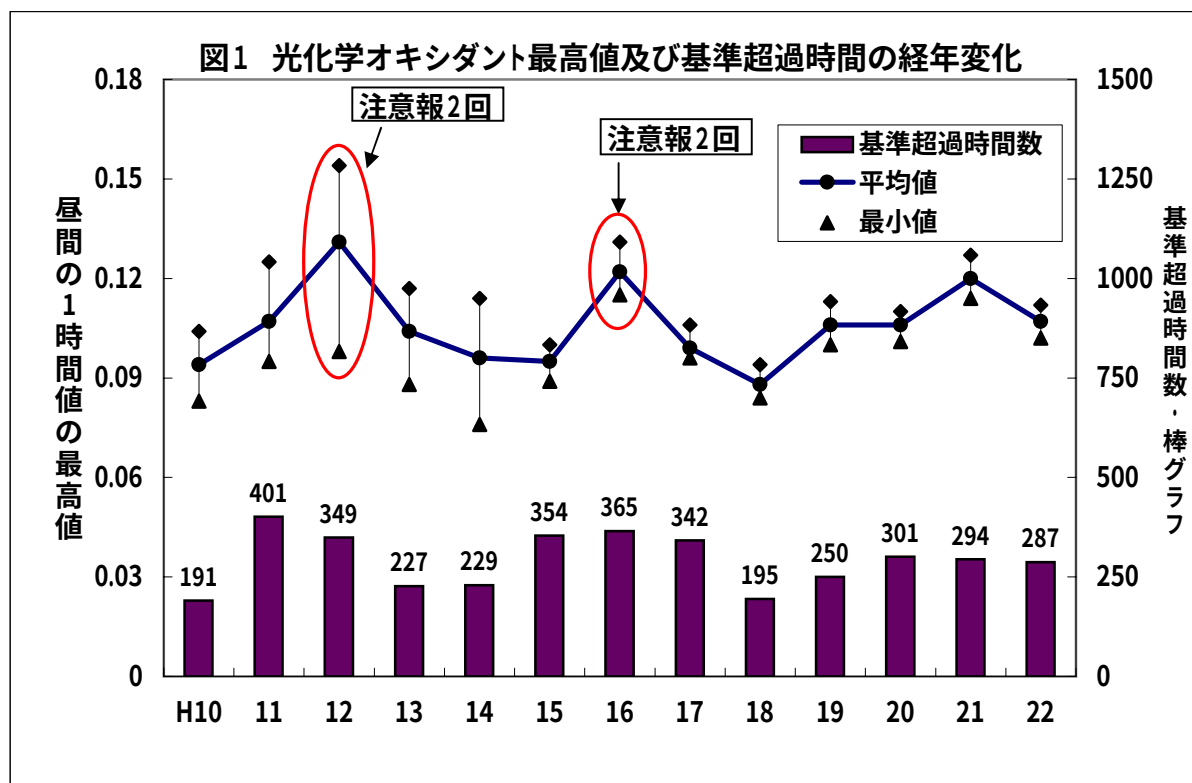
図2 光化学オキシダントの環境超過時間数と最高濃度の推移
