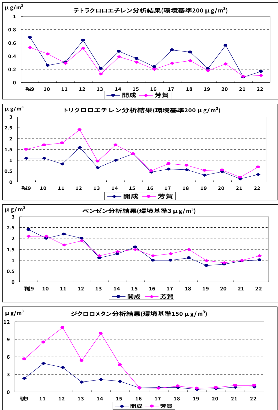
図1 有害大気汚染物質の推移
