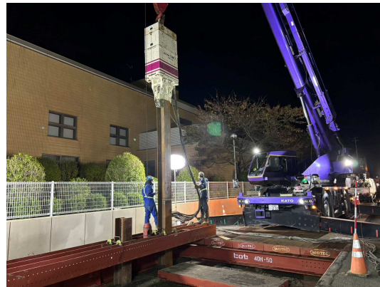
親杭設置状況
