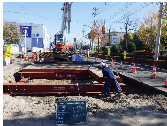
覆工板設置状況
