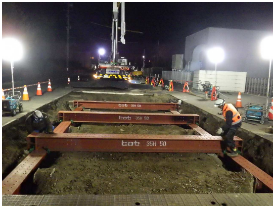
桁受設置状況
