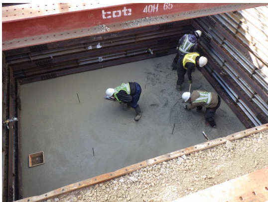
特殊人孔基礎コンクリート打設状況
