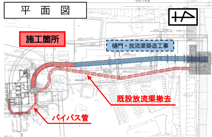
バイパス管布設状況
