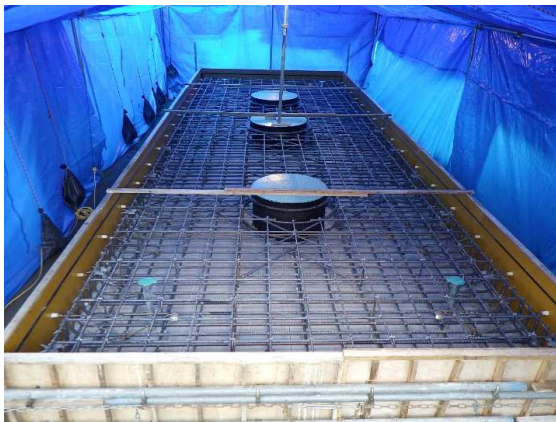
地下オイルタンク頂版鉄筋組立完了
