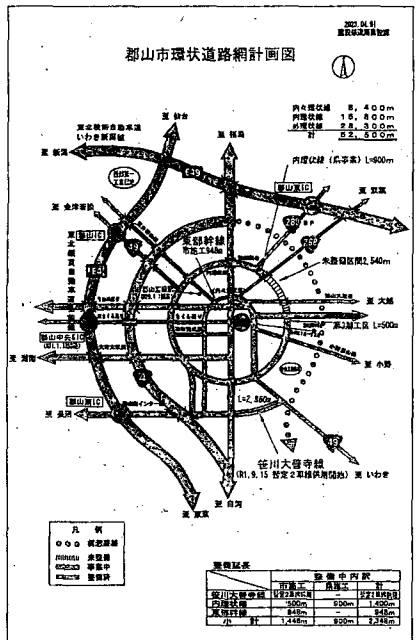
郡山市環状道路網計画図
