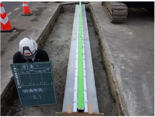
排水構造物(円形側溝)設置状況
