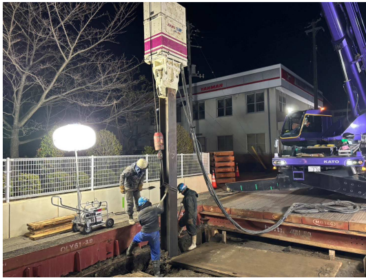
親杭(H鋼)・横矢板引抜き状況
