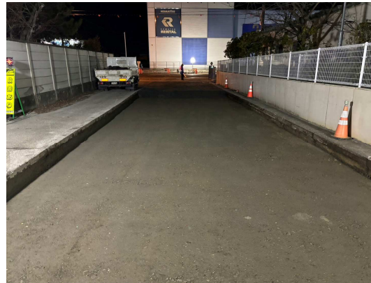
路盤転圧完了
