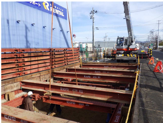
切梁・腹起し設置状況
