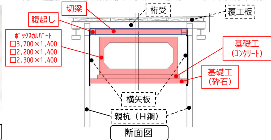
ボックスカルバート布設完了
