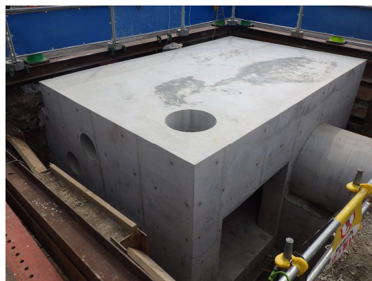
特殊人孔 設置完了
