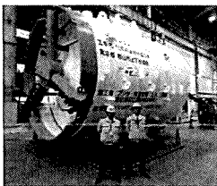
図案貯留管 (直径4,530mmのシールド掘進機)
