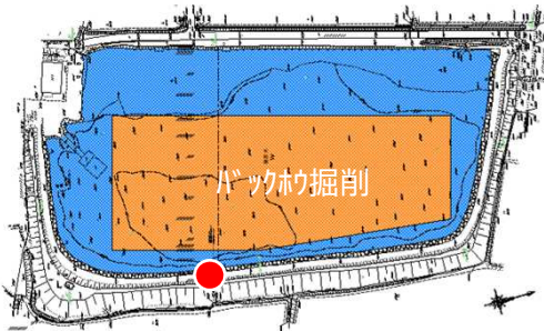
対策計画図
