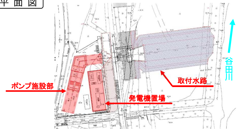
平面図
