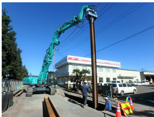
親杭設置状況（土留工）
