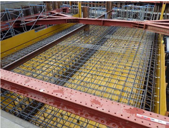
ポンプ施設部鉄筋組立完了
