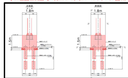
基礎構造図
