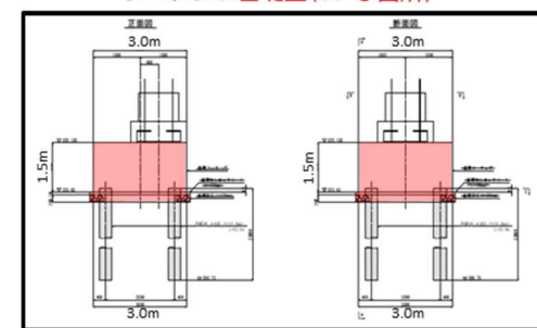
基礎構造図
