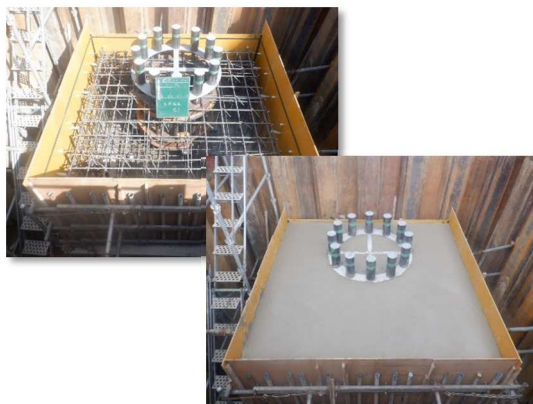
フーチング基礎工施工状況(S-P1)
