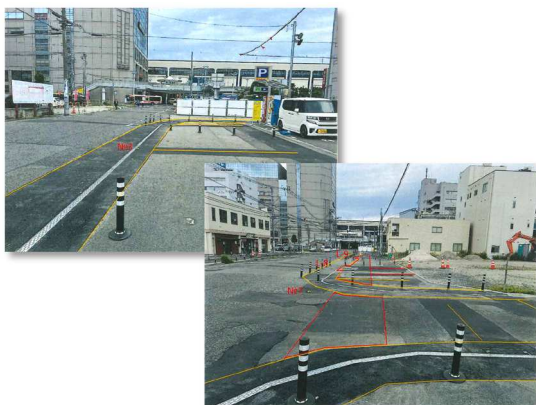
電線共同溝等施工完了状況(東側を望む)
