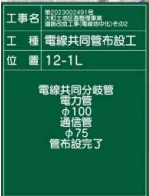
電線共同溝(管路部)施工状況
