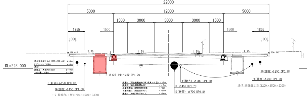
標準横断面
