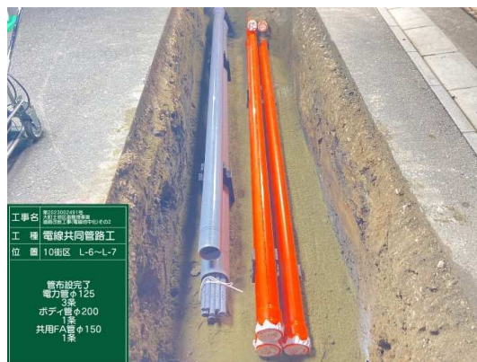
電線共同溝(管路部)施工状況
