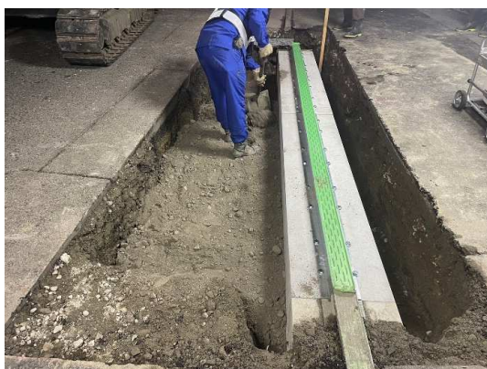
円形側溝設置状況
