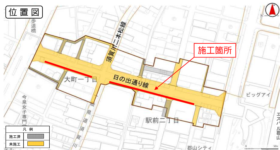
電線共同溝(管路部)施工状況
