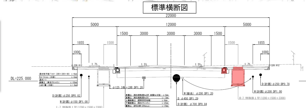
排水構造物(円形側溝)設置状況
