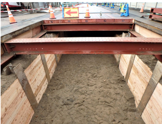
桁受・受桁設置完了（土留工）
