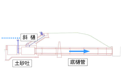
放流施設 計画図
