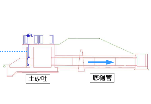
放流施設 計画図
