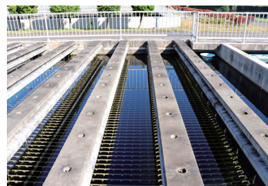
薬品沈でん池
