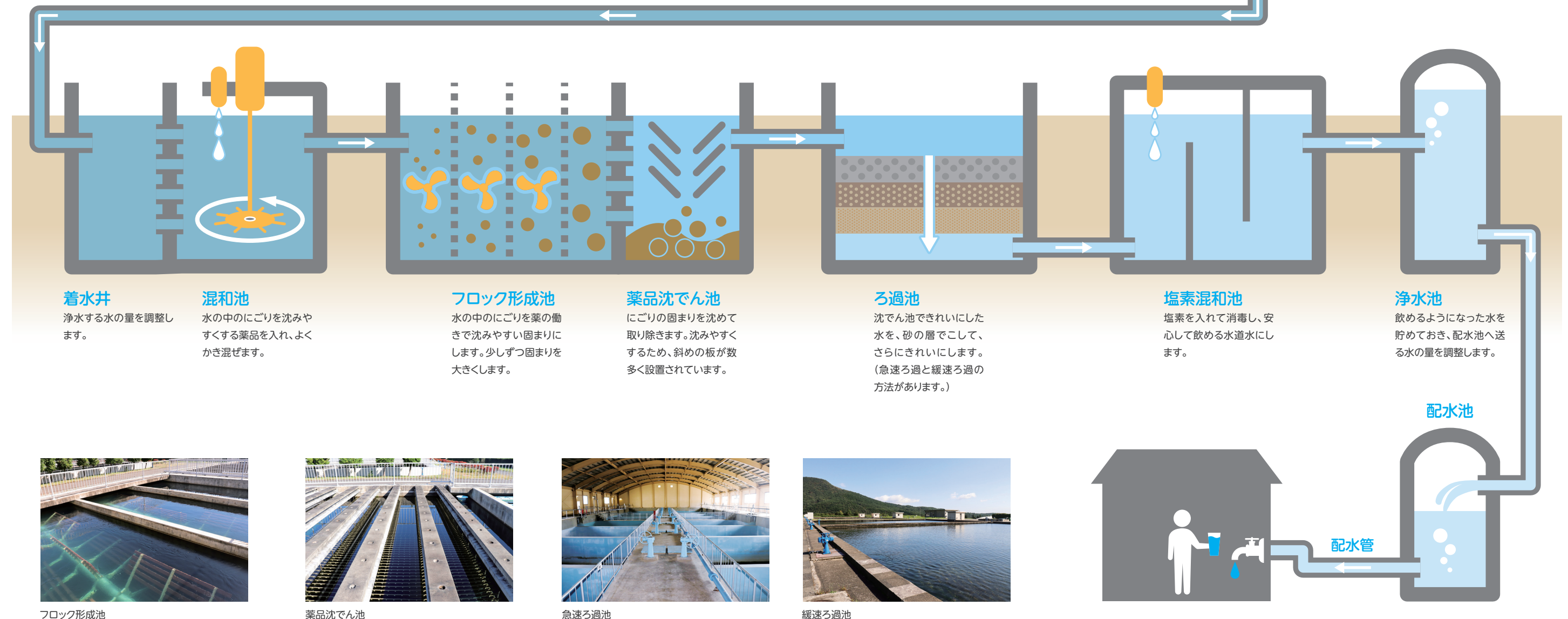
フロック形成池
